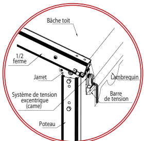
Tension toit
