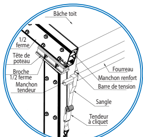
Tension toit
