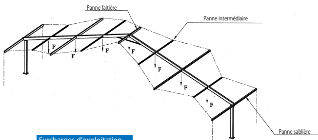
Surcharges d'exploitation
